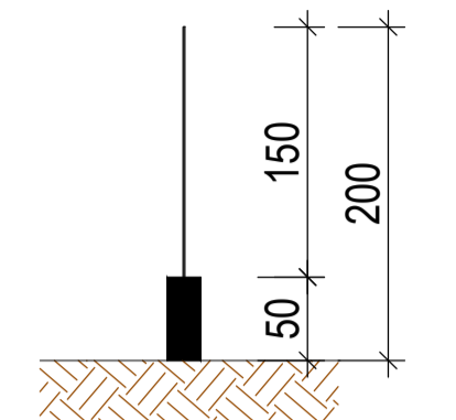
SEZIONE TIPO A
