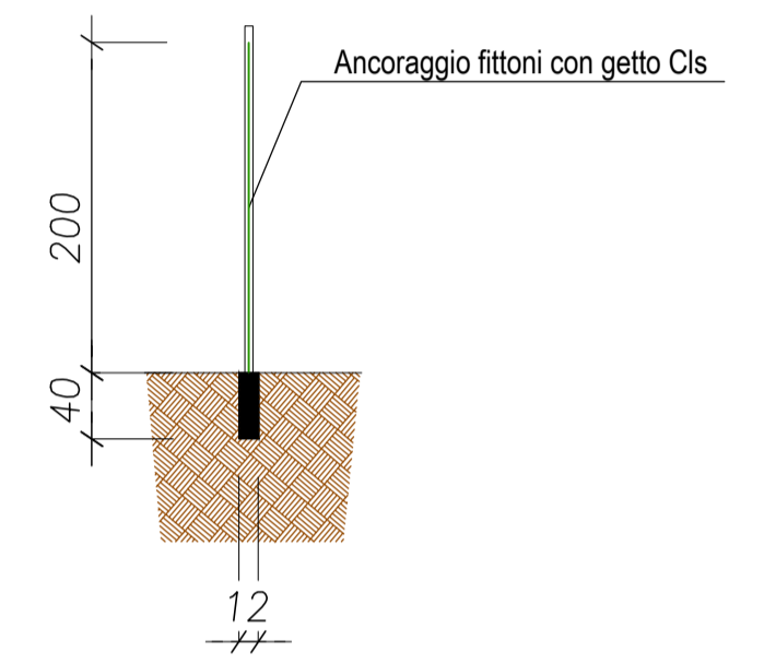
SEZIONE TIPO B
