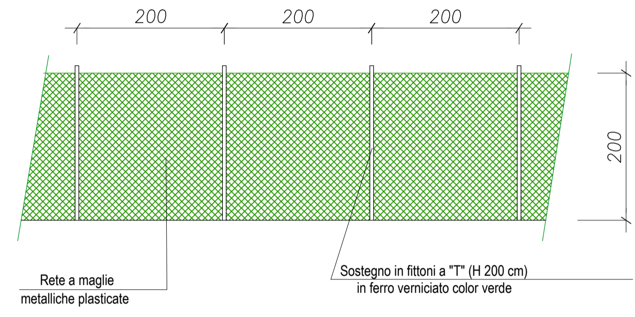
PROSPETTO TIPO B
