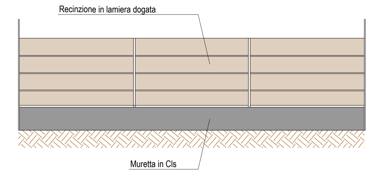
PROSPETTO TIPO A
